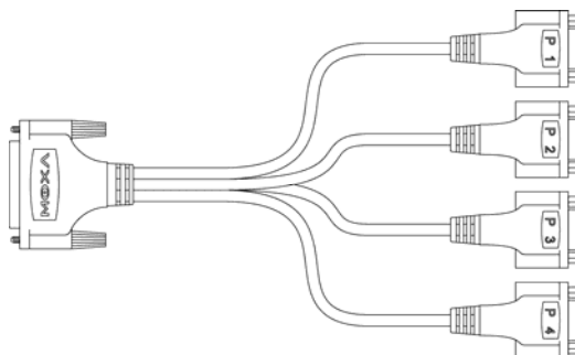
Модель CBL-M44M25x4
