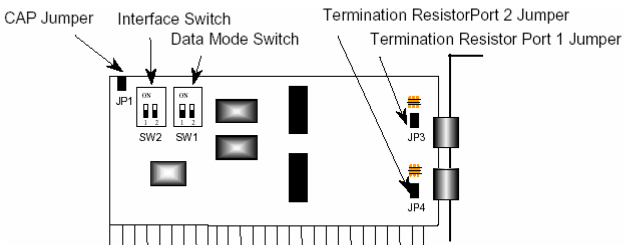
Плата серии Industio CI-132
